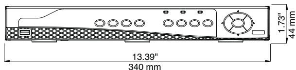
Voor aanzicht
